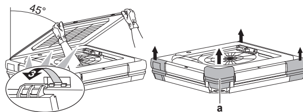
a Кутова кришка
