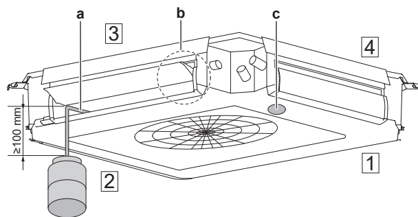
a Пластикова ємність для води з трубкою довжиною \geq 100 mm b Дренажний насос і розташування поплавкового реле c Отвір для зливу при обслуговуванні (з гумовою пробкою). Використовуйте цей отвір для зливу води з лотка для конденсату.
