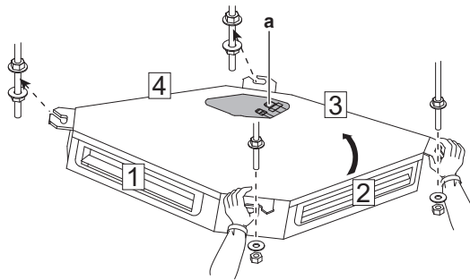
a Деталь трубопроводу
