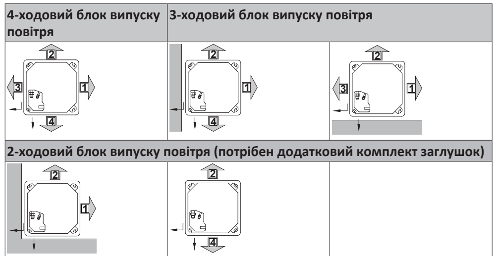
16-1 Схема випуску (вид згори)
