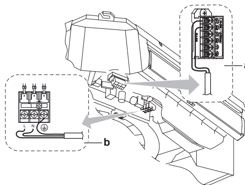
a Клемний блок пульта користувача b Клемний блок джерела живлення
