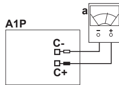
A1P Головна печатна плата a Мультиметр C Точки вимірювання залишкової напруги
