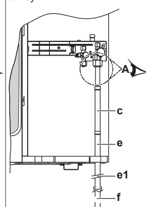
Вариант 4: подсоединение снизу
